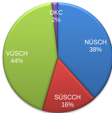
AVNRT
